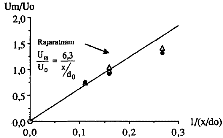
Fig. 6. Décroissance axiale de la vitesse du gaz dans le jet. Cas de la colonne vide.
